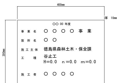
図1 銘板の寸法及び記載事項
